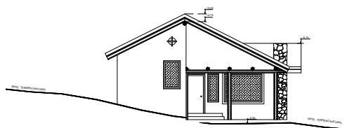
ELEVACION PONIENTE
