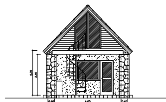
ELEVACION PONIENTE
