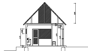
CORTE A - A
